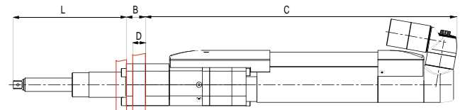
СТ – прямая модель
