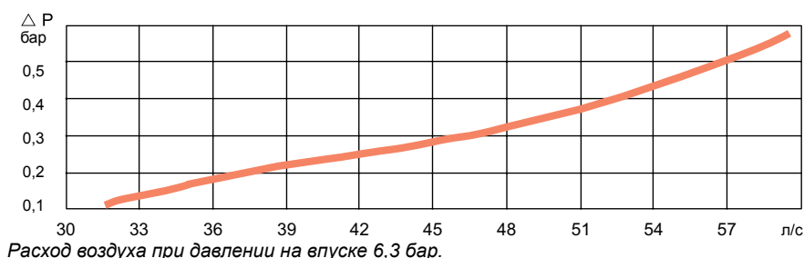
График. QIC 15SE M15 и NIP 15E F15
