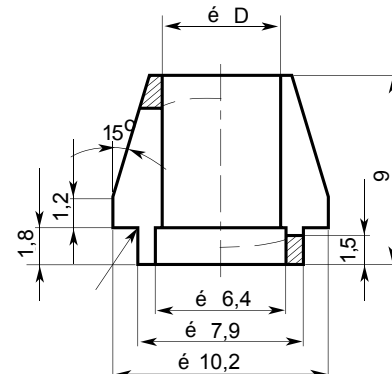
Цанговые патроны для головок с макс. диам. сверла 6,6 мм
