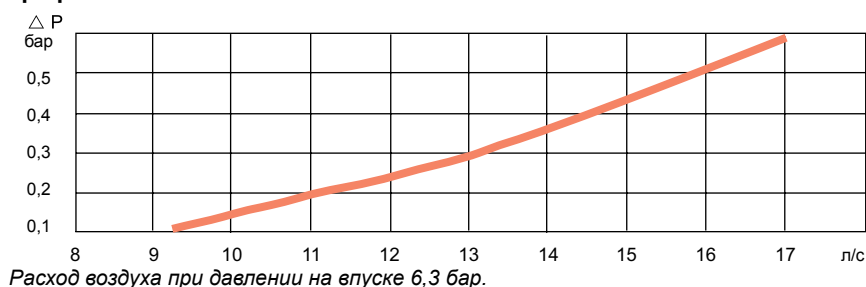
График. QIC 08 M08 и NIP 08 F08
