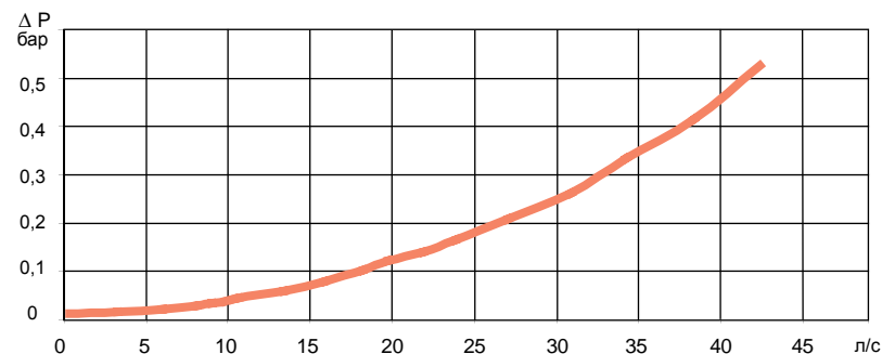
График. ErgoQIC 10US и NIP 10US
