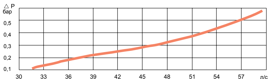
Расход воздуха при давлении на впуске 6,3 бар.
