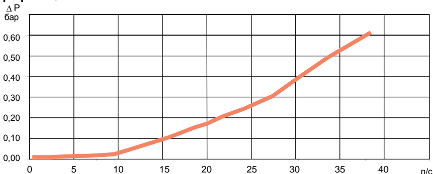
Расход воздуха при давлении на впуске 6,3 бар.
