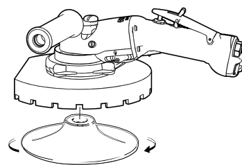
Комплект всасывания (для зачистки волокнистым кругом)
