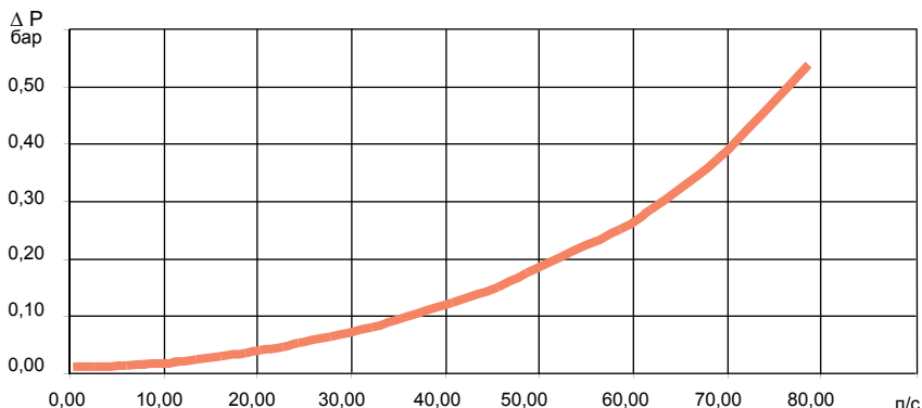
Расход воздуха при давлении на впуске 6,3 бар.
