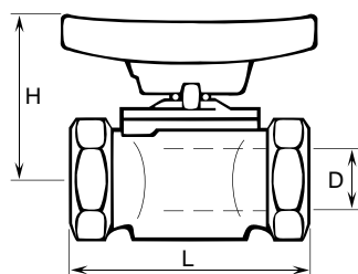
Двойное соединение
