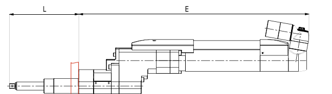
COT – модель со смещенным редуктором
