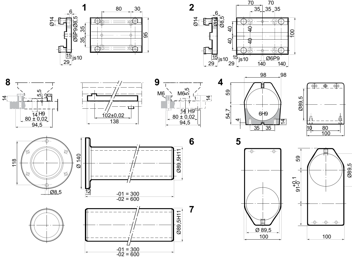
Чертеж с размерами – крепления для LBL45E
