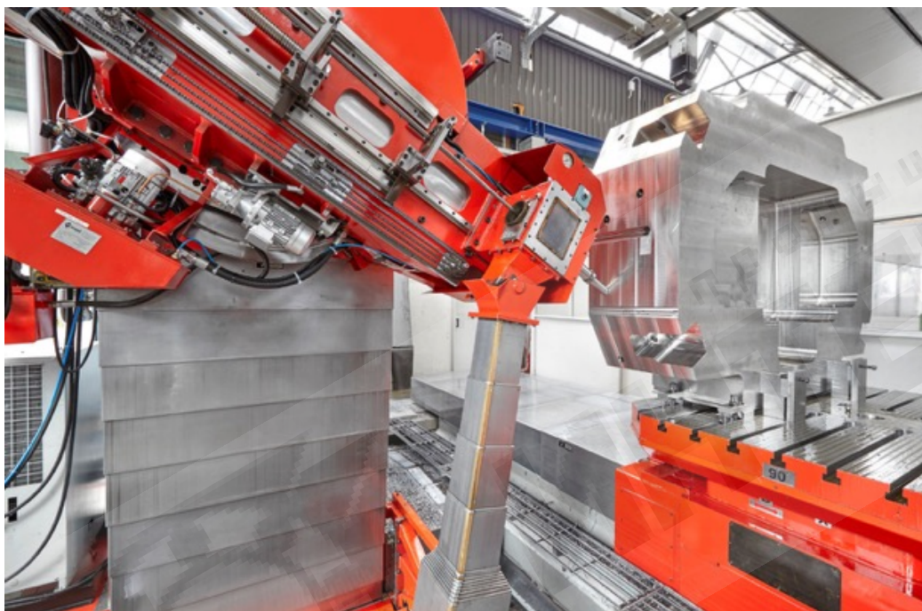
Сверлильный станок для глубоких отверстий
