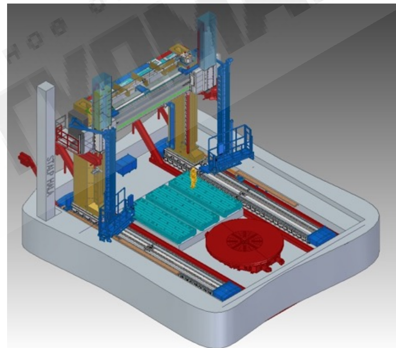
Вертикальный токарный станок - Ø 8500 мм
