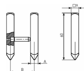
Разметочные губки
