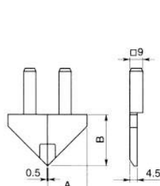
Стандартные губки
