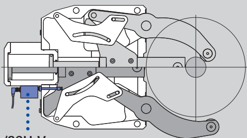
SCU-A/SCU-V
